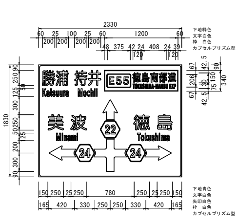
121 案内・予告標識 (1830x2330) 板交換
