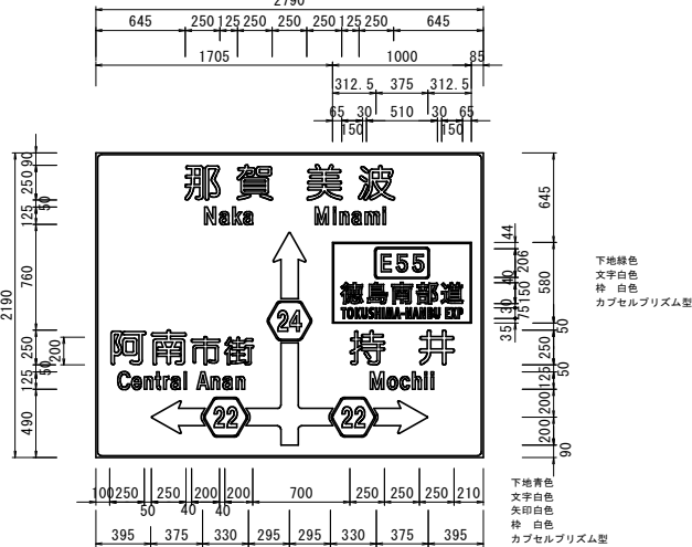
125 案内・予告標識 (2190x2790) 建て替え
