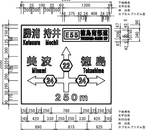
120 案内・予告標識 (2050x2330) 板交換
